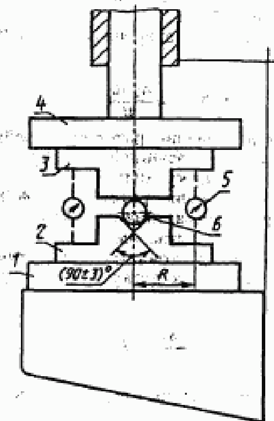
1 и 4 — плиты; 2 и 3 — стальные призмы; 5 — индикатор; 6 — шарик
